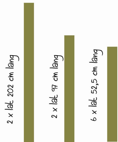
Latten voor frame dak
