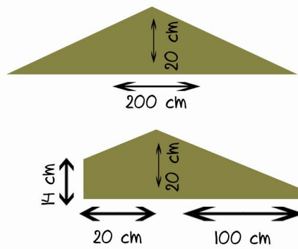
2 x plaat voor- en achterzijde dak
