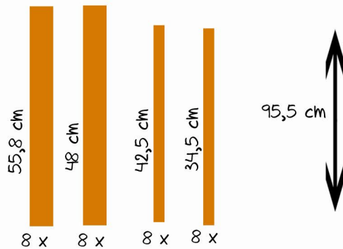
32 x latten kozijnen
